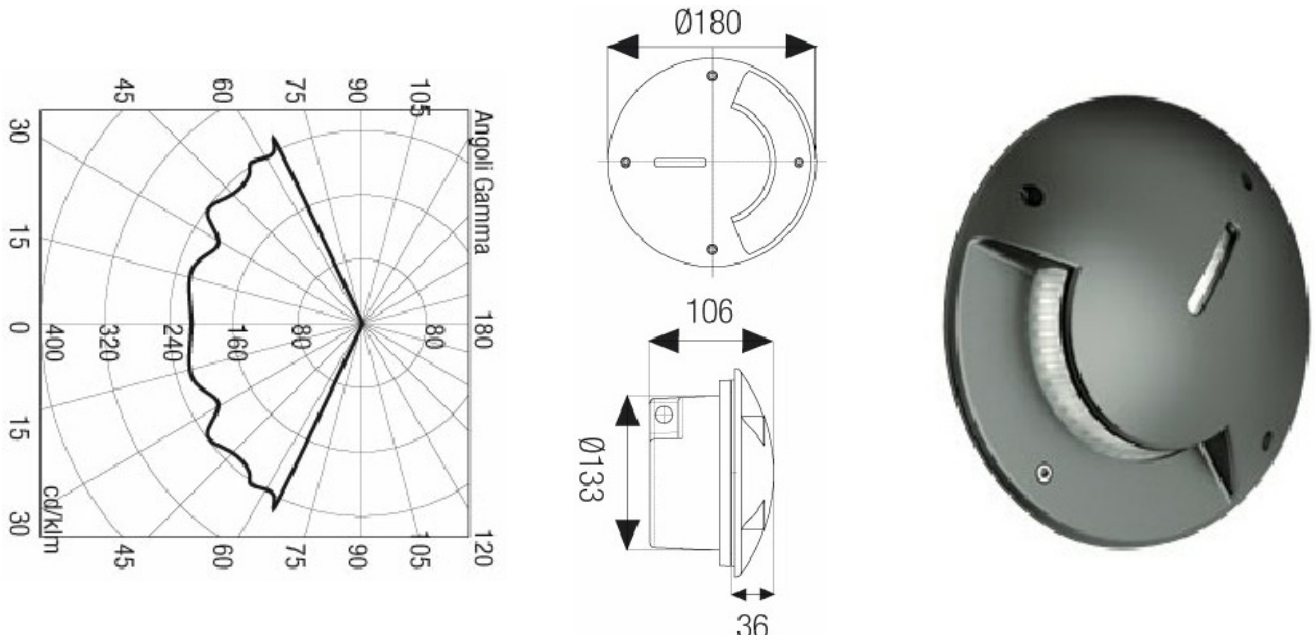
PUNTO LUCE TIPO SEGNAPASSO
